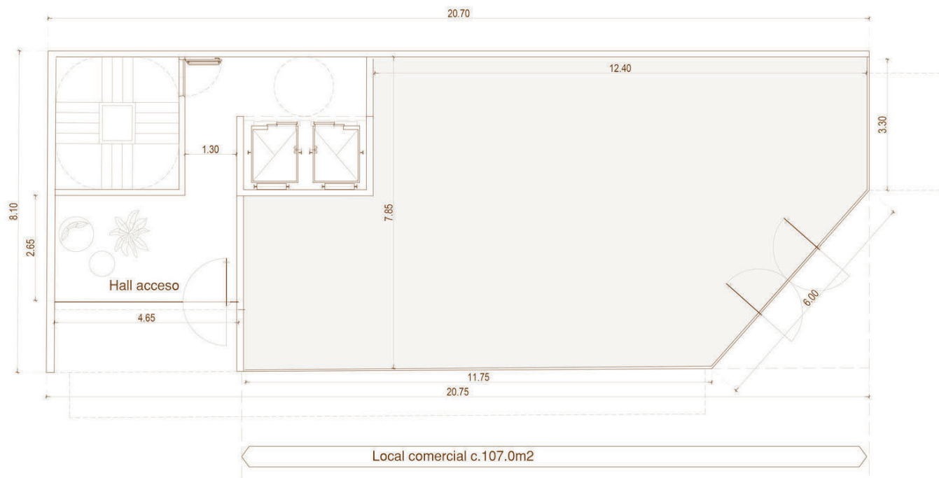
PLANTA BAJA Esc. 1/75
